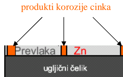
Slika 6. Anodna prevlaka cinka na željezu [10]
