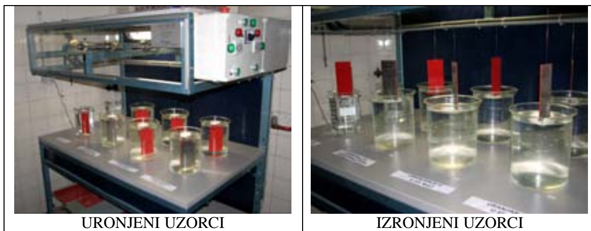
Slika 34. Položaji uzoraka tijekom ispitivanja uranjanjem [29]
