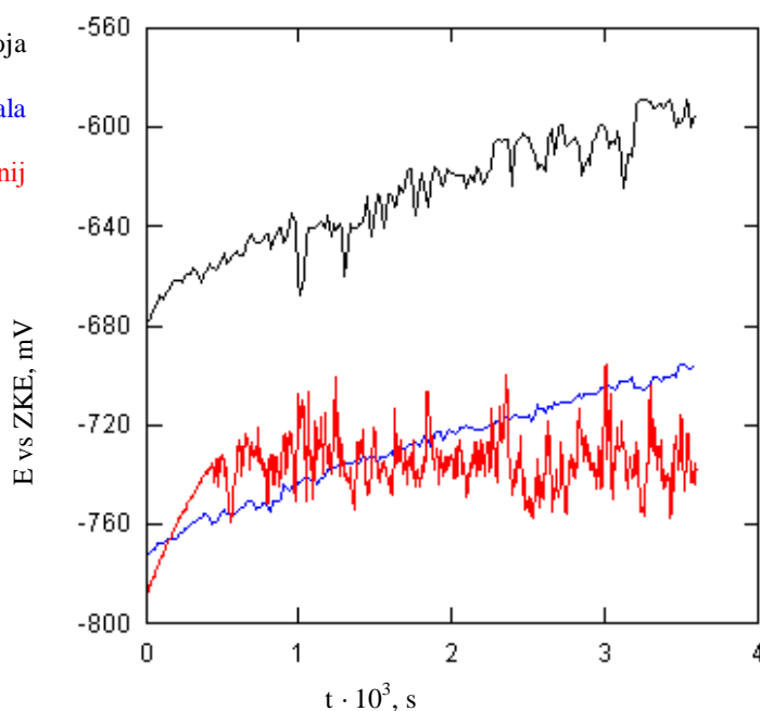
Slika 45. Dijagram E_{kor} - t za aluminijske uzorke
